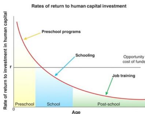
Slika 1: Heckmanova krivulja
